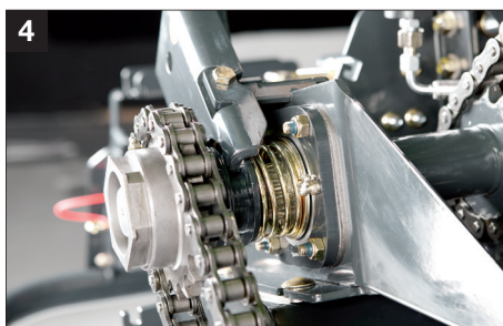
Механическое отключение ротора
