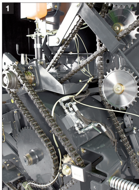
Простой привод с устройством защиты кулачковой муфты
